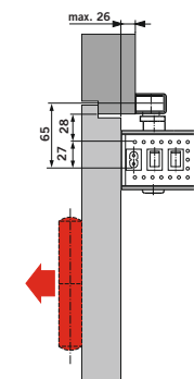
Türblattmontage auf der Bandgegenseite
