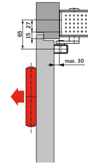
Sturzmontage auf der Bandgegenseite
