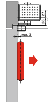
Sturzmontage auf der Bandseite
