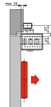
Türblattmontage auf der Bandseite
